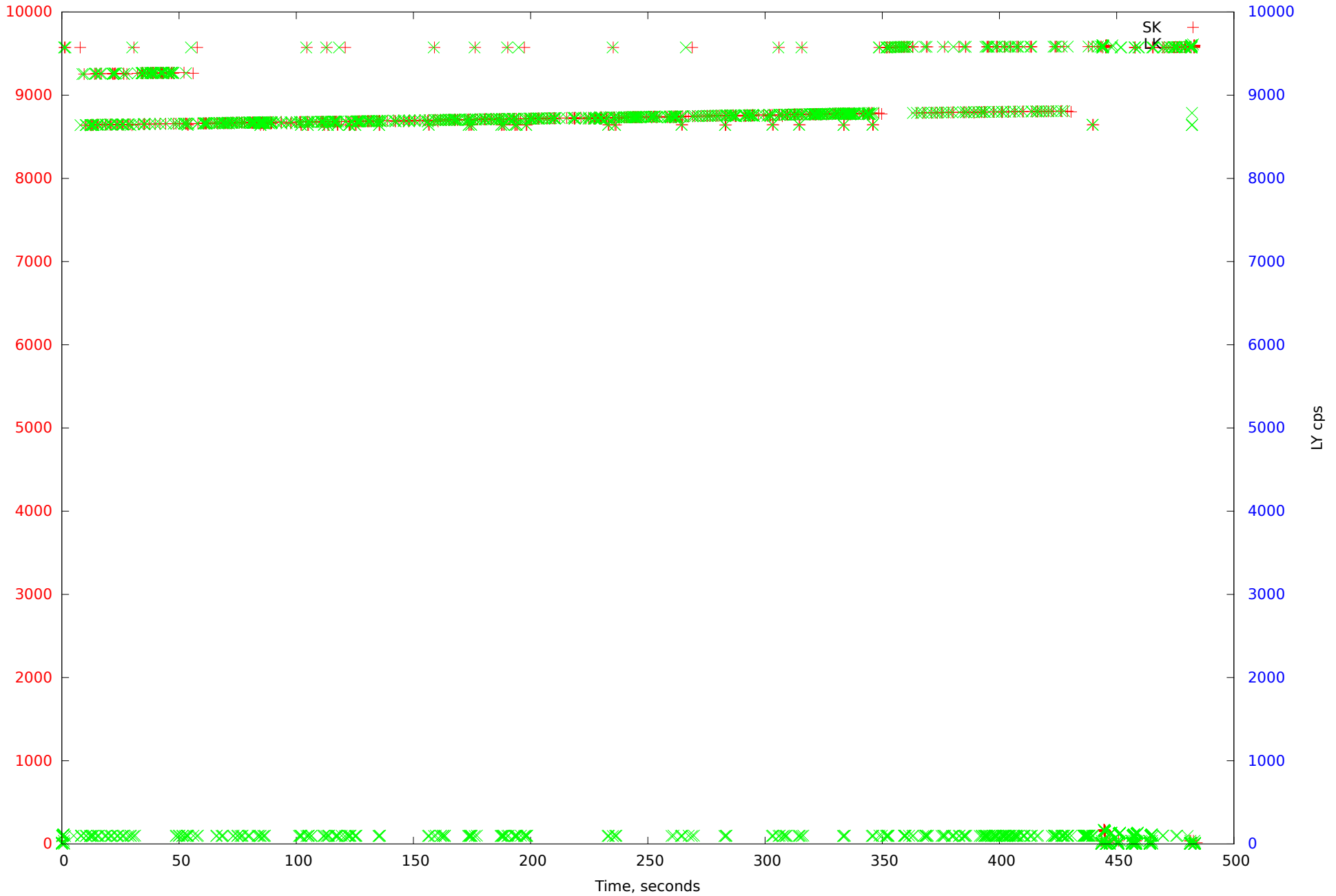
gier.debug.2
